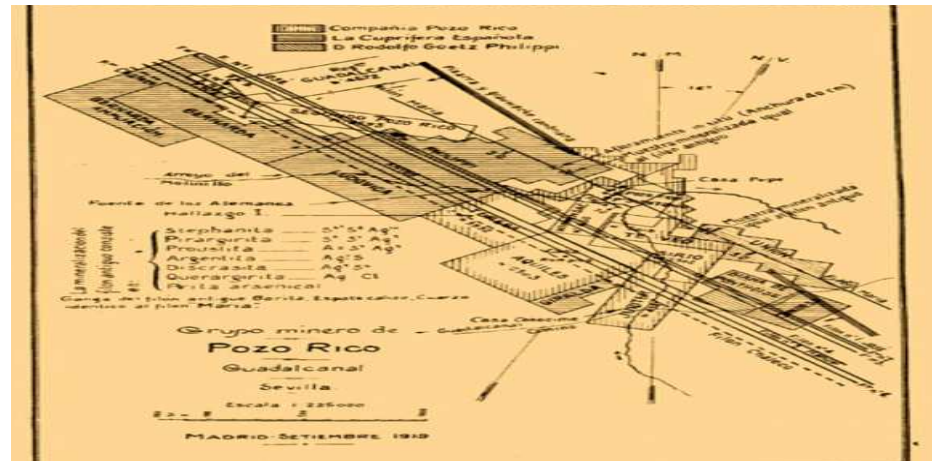
Plano de la minas de Pozo Rico
